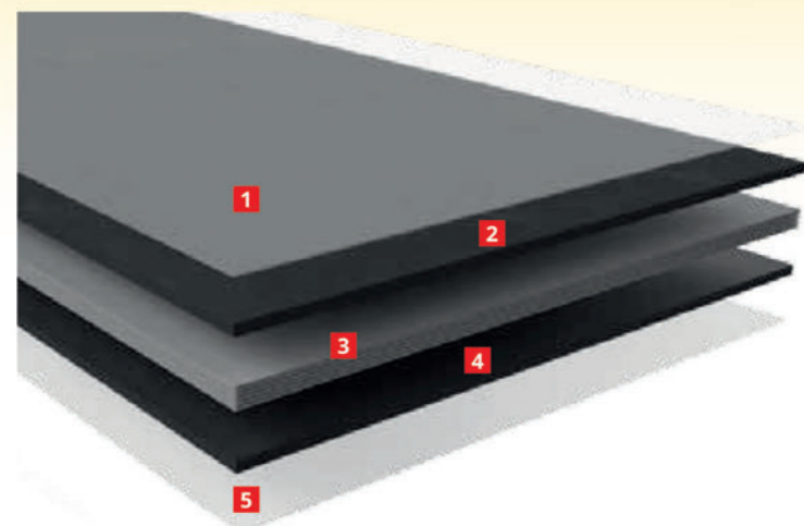
1 Schutz-Overlay | 2 Dekorpapier | 3 Kern - Kraftpapiere (Phenolharz) | 4 Dekorpapier | 5 Schutz-Overlay
